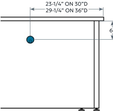
Grommet on U-Shape Table
